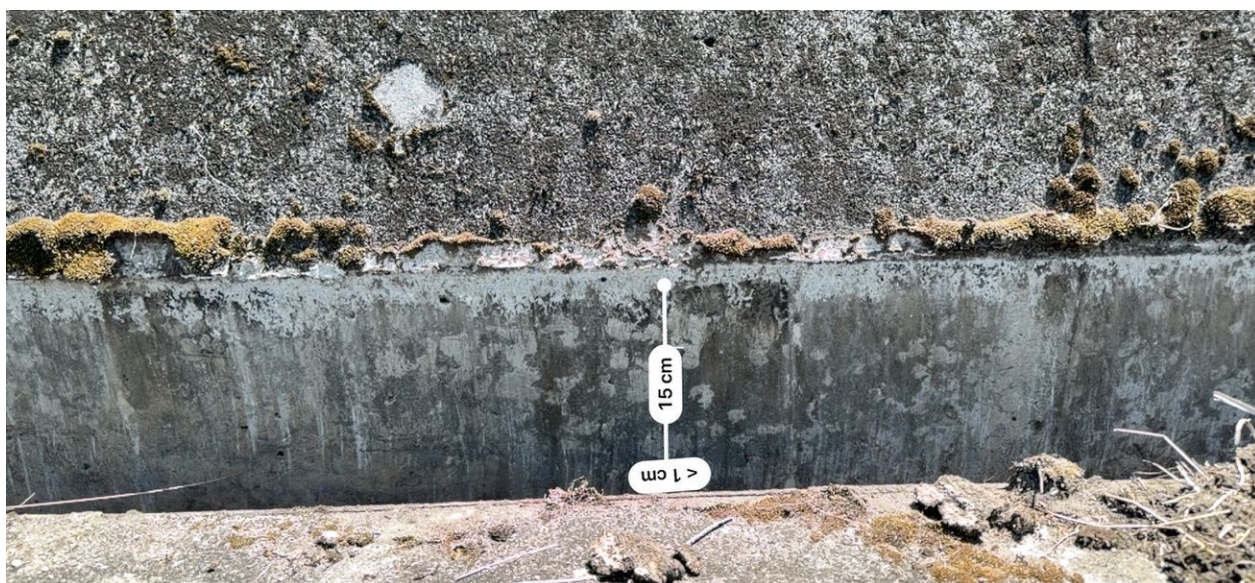
写真 2 1. 堤防にひび割れと変形が発生した。
